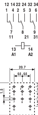
Csatlakozók nézetei
