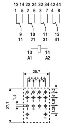
Csatlakozók nézetei
